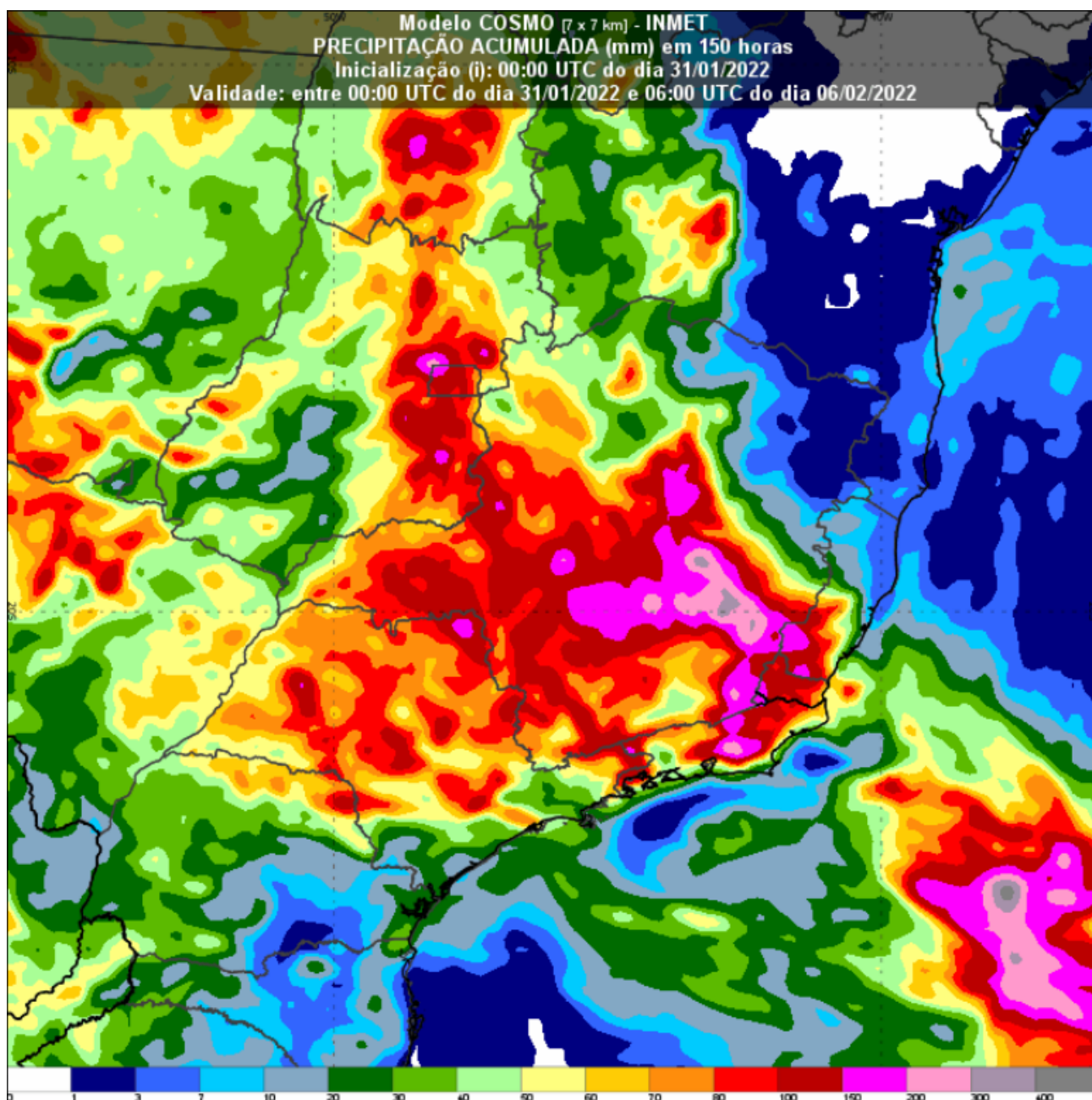
Figura 1 – Simulação do modelo COSMO/INMET com o acumulado dos próximos dias.
